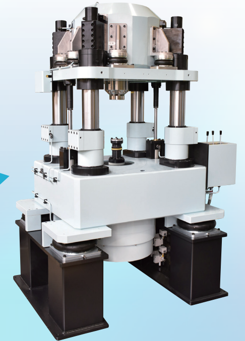
弹性体动态特性试验机
